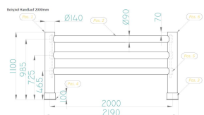
Technische Zeichnung Handlauf
