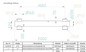
Technische Zeichnung Rammschutzbarriere Einzelplanke
