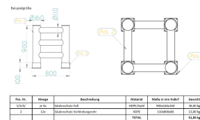
Technische Zeichnung Säulenschutz Strong
